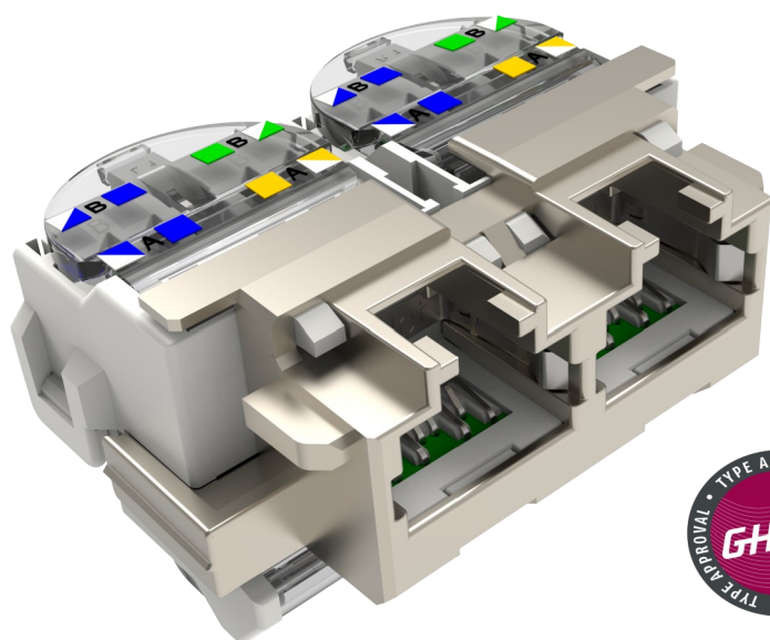
Abb. 1: Ansicht von vorne
