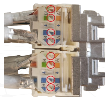
Abb. 3: Sichtkontrolle nach Beschaltung durch integrierte Sichtfenster
