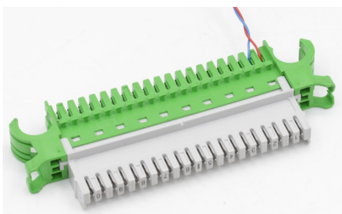
Abbildung 3: ohne Zugentlastungskamm
