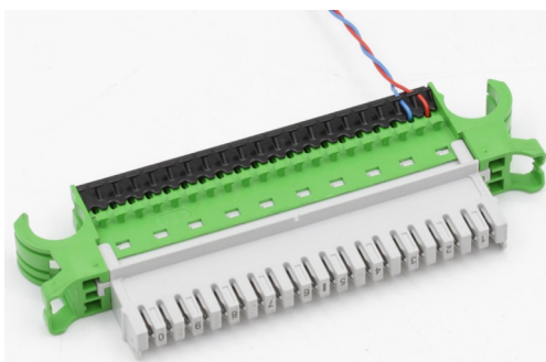
Abbildung 2: mit Zugentlastungskamm
